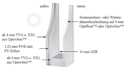
Zweiseiben-Isolierglas mit Pilkington Sunplus™ BIPV
