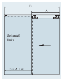
A Glasbreite, B Laufschienenlänge,
